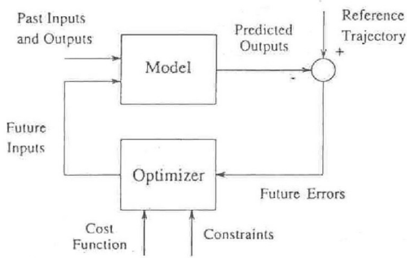
شكل 6.3: مخطط صندوق يظهر كيف يتم تطبيق التحكم التنبؤي
