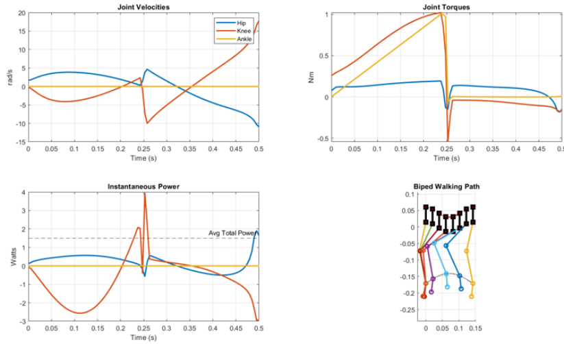
شكل 3.5: العزوم والسرع والطاقة المسحوبة من الرجل عند تطبيق مسار حركة المشي
